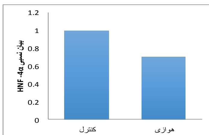
نمودار ۴. بیان نسبی HNF-4 \alpha در گروه‌های هوازی و کنترل پس از دوره تمرین
